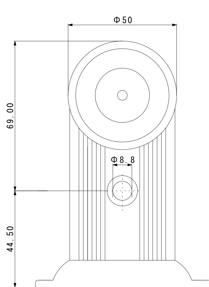
【RESCR-SKX5EHM 寸法図】【本体】
